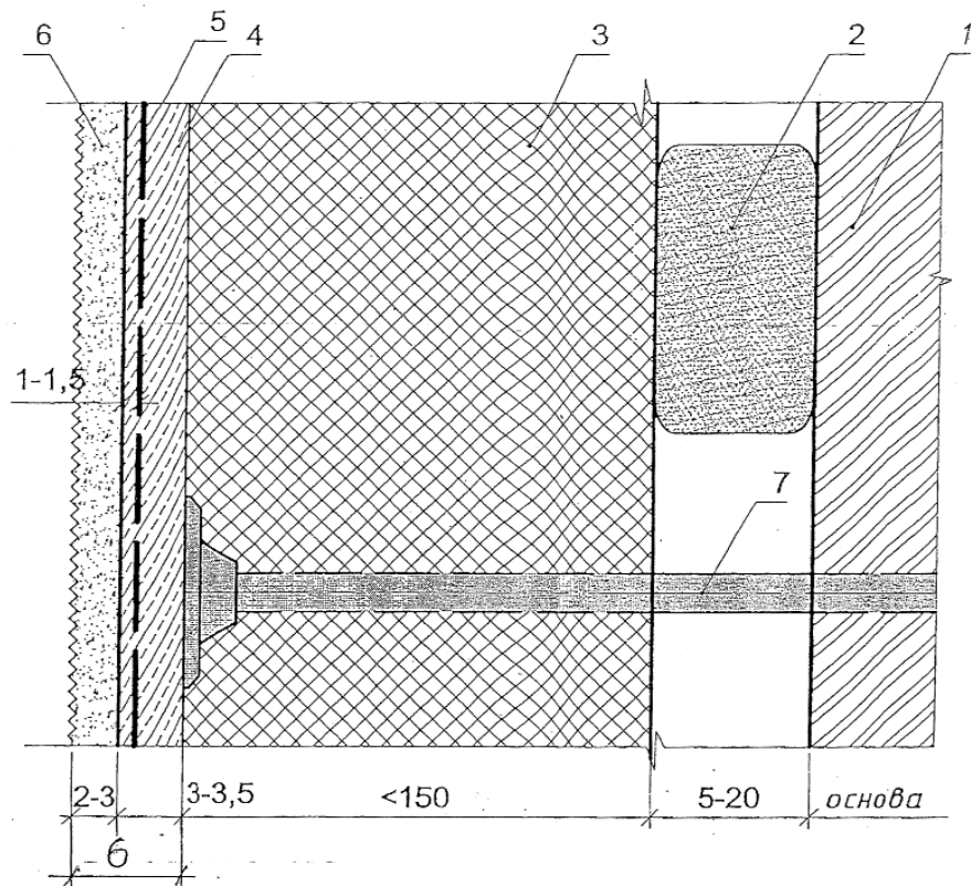
Рис. 1. Конструктивно-технологічне рішення системи класу А: 1 – основа; 2 – клейовий шар; 3 – утеплювач; 4 – матричний шар; 5 – скосітка; 6 – захисно-опоряджувальний шар; 7 – дюбель.
